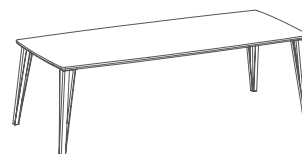
GO.TA240FIX 240 x 98 x 75 cm
